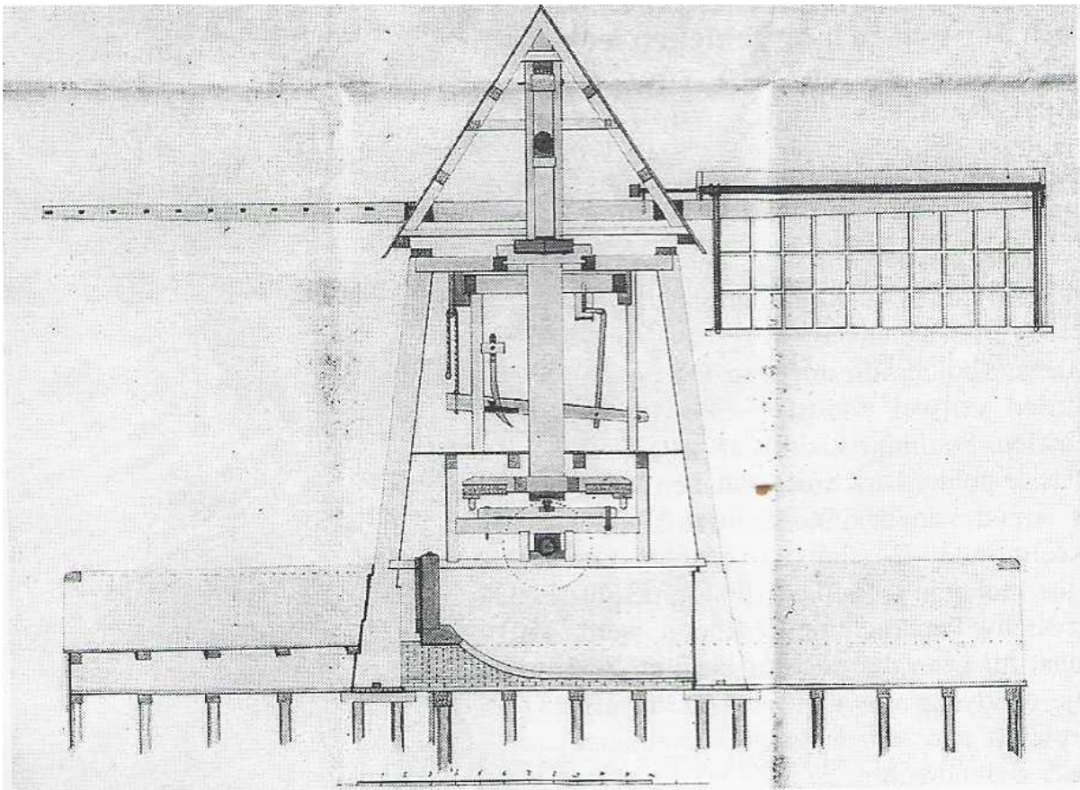
Tekening van "een horisontale scheprad watermolen" in de Lakerpolder (Algemeen Rijksarchief Den Haag).
