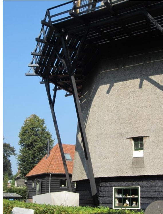
Afb. 12 De (lange) schoren – met kraaienpoten – steunen onderaan op de achtkantstijlen, waardoor geen ondersluiting nodig is. Het zijn bijna stutten ... (De Zandhaas – Santpoort)
