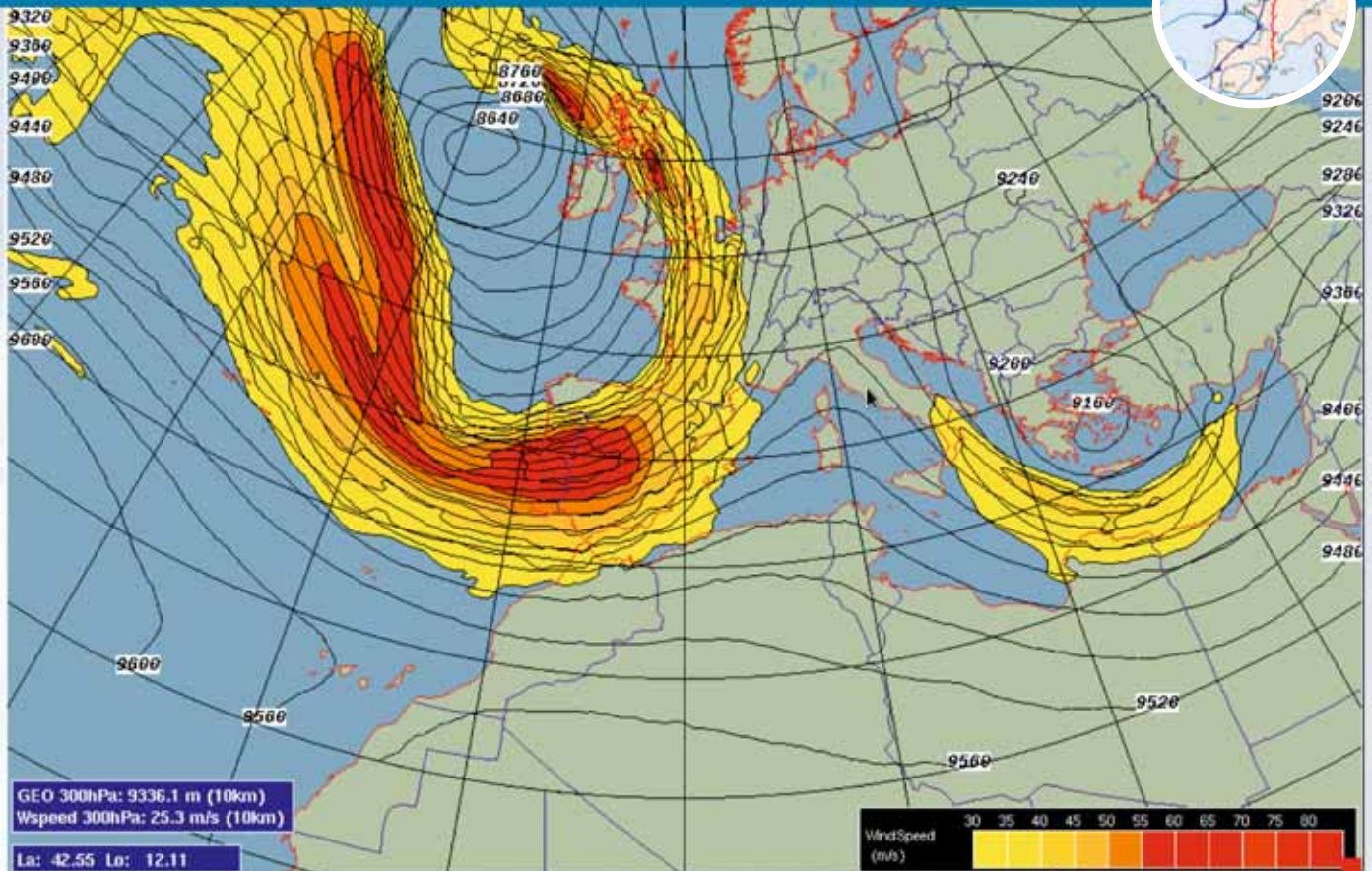
Afb 1. Een kronkel van de straalstroom ligt over Spanje via Schotland naar IJsland. In de as komen windsnelheden voor 80 meter per seconde ofwel 288 kilometer per uur. Dit is een kaart van de luchtdruk op 9,3 kilometer hoogte.
