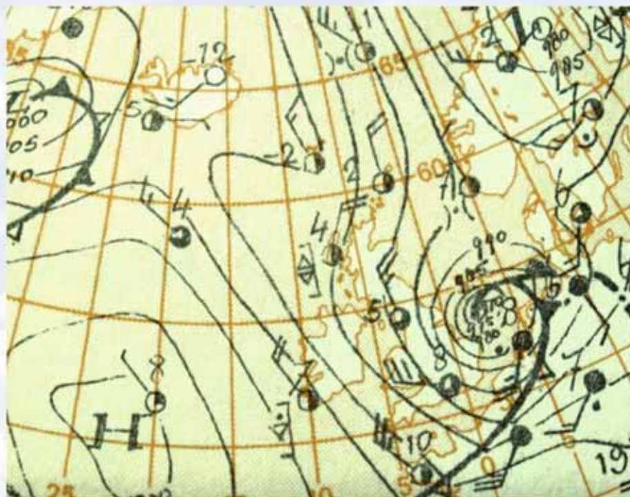
Afb 3. Een weerkaart van 2 april 1973. Een van de zwaarste stormen ooit, veroorzaakt door een 975 hPa diep lagedrukgebied. De isobaren liggen dichtbij elkaar, goed voor een korte maar hevige zeer zware storm.
