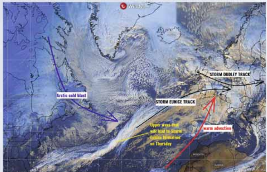
Afb 2. Op de satellietfoto is goed te zien hoe zuidelijk de Canadese winterkou de Atlantische Oceaan op trekt. Dit gebeurt niet alleen aan de grond maar ook op grotere hoogte.
