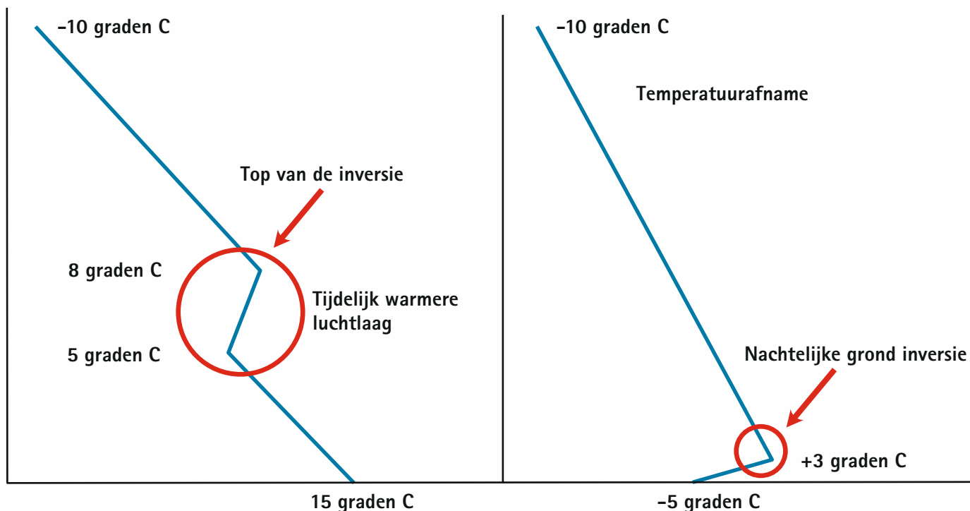
Afb 1. Voorbeeld van twee inversies. Aan de linker kant zie je een tijdelijk warmere luchtlag op enige hoogte in de lucht. Aan de rechter kant zie je een inversie aan de grond, de meest voorkomende vorm van een inversie. (Eigen tekening)
